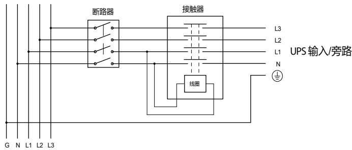
三相输入系统示意图
