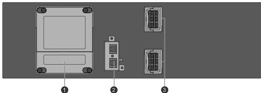
PTB 9161 电池箱
