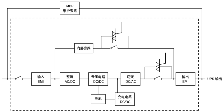
系统框图
